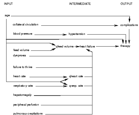
Figuur 3.8: Combinatie van expertise- en taakmodel: afhankelijkheidsnetwerk.
