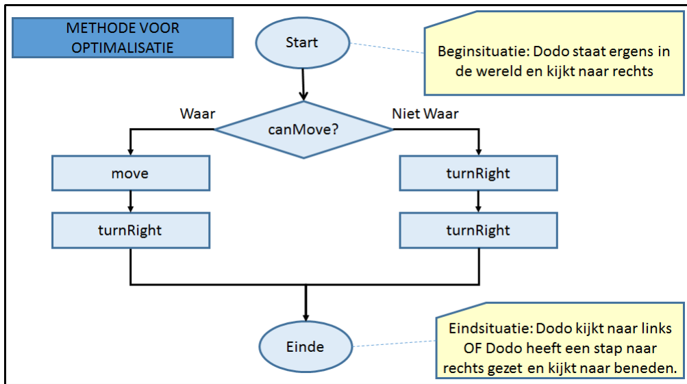
Figuur 4: Stroomdiagram vóór optimalisatie
